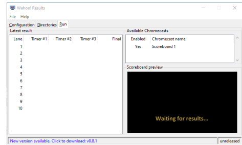
Fig. 5: Run tab
