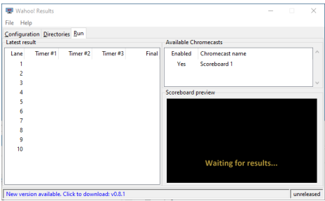
Fig. 5: Run tab
